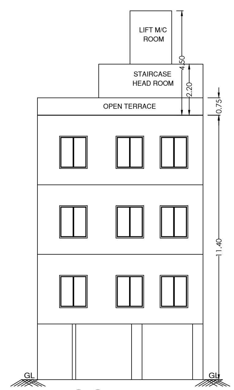
ELEVATION
